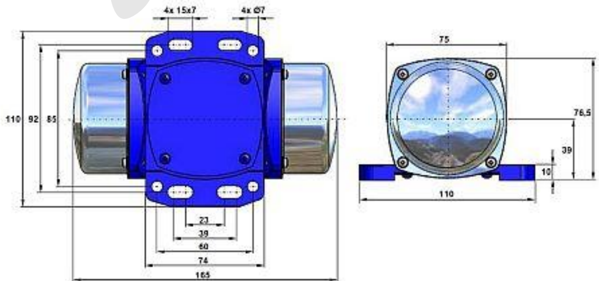
Abbildung 2 Abmaße
