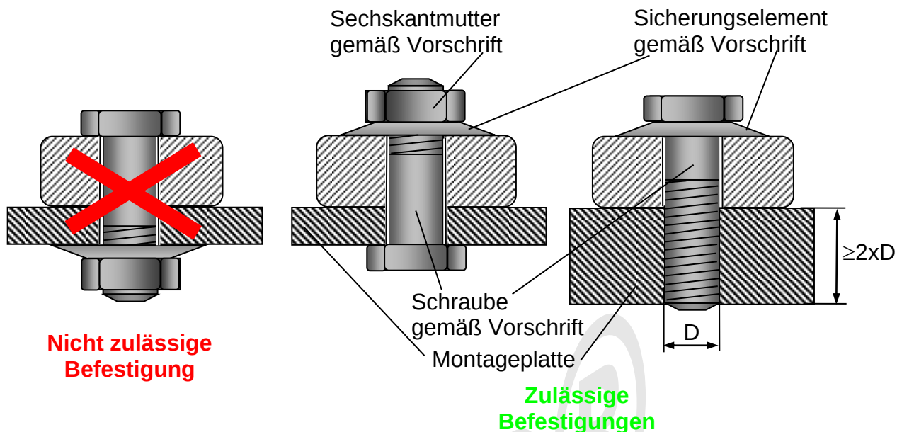
Abbildung 3 Befestigungsarten des Rüttelmotor
