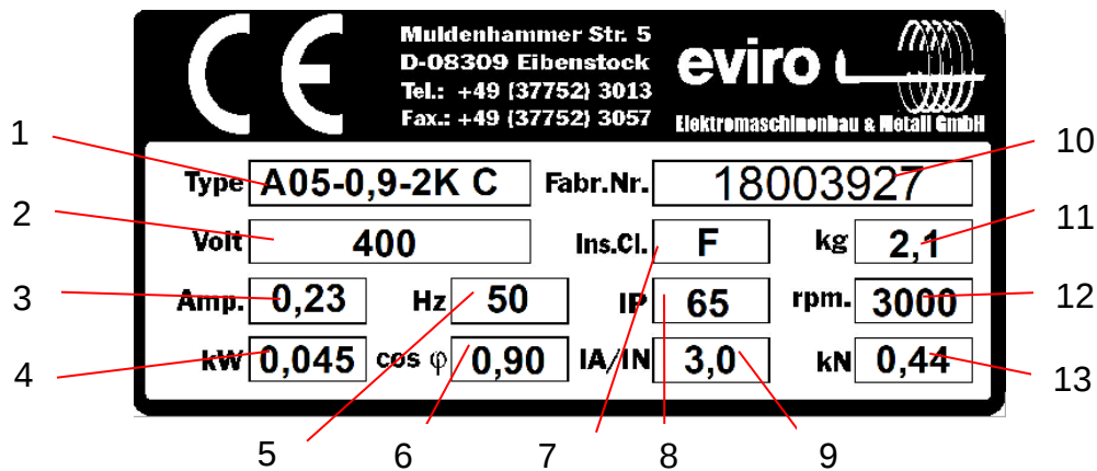
Abbildung 1 Typenschild
